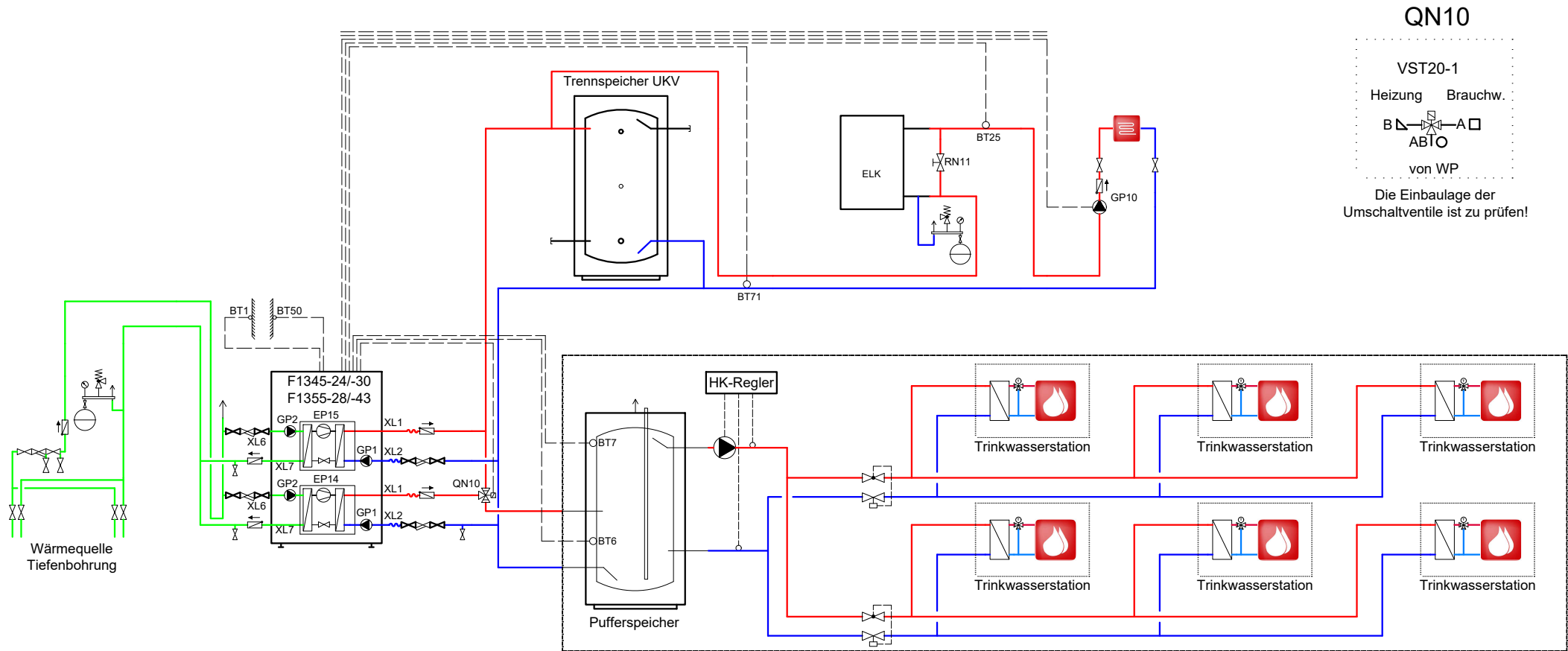
Dies ist eine Beispielhydraulik. Der Anschluss muss nach Vorgaben des Herstellers der Trinkwasserstationen erfolgen.
