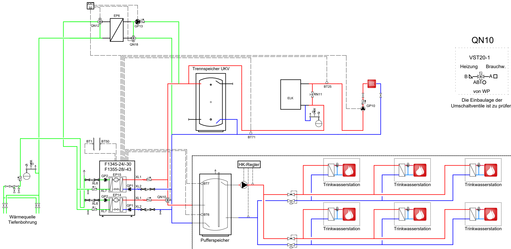
Dies ist eine Beispielhydraulik. Der Anschluss muss nach Vorgaben des Herstellers der Trinkwasserstationen erfolgen.
