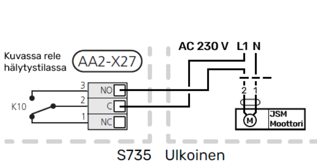
AUX lähdön (AA2-X27) sijainti S735 poistoilmalämpöpumpussa
